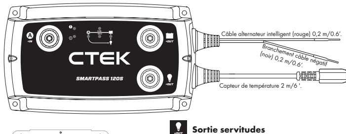
Plaque de connexion
